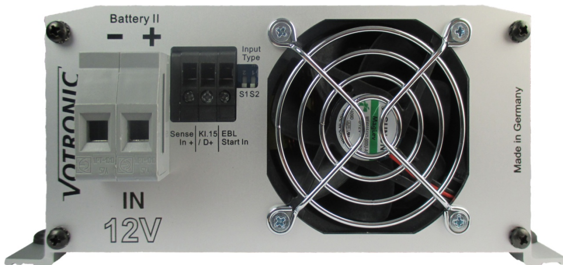
Ansicht Frontplatte Eingang
