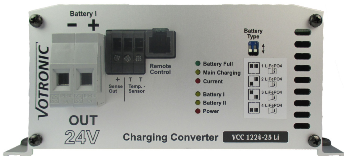
Ansicht Frontplatte Ausgang
